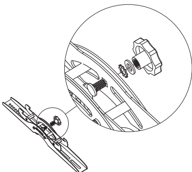
(6)M8x90 Wandschraube-u
